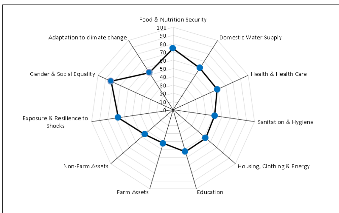
MPAT (2014) Subcomponents
